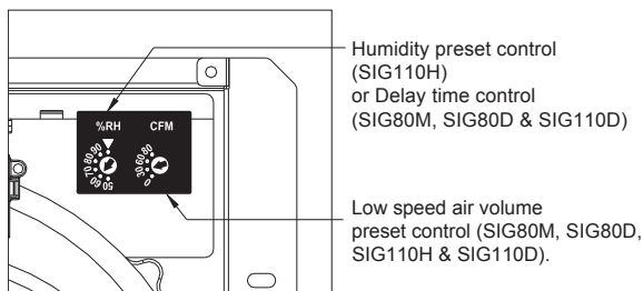
SIG110H control options
